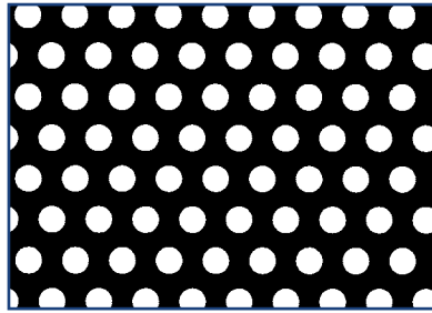
UML 102
