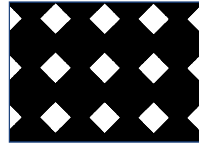
UML 116
