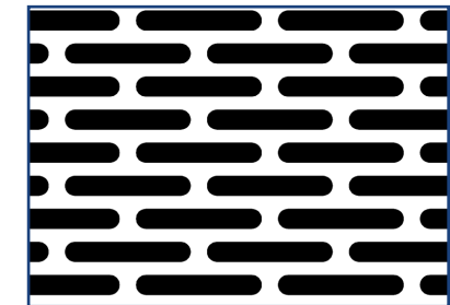
UML 127
