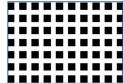
UML 124
