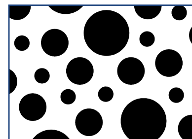
UML 128
