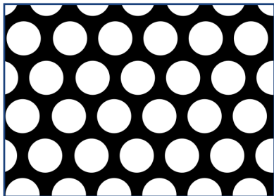
UML 107
