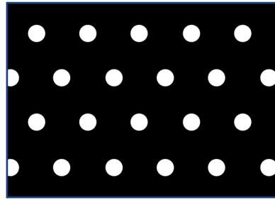
UML 103
