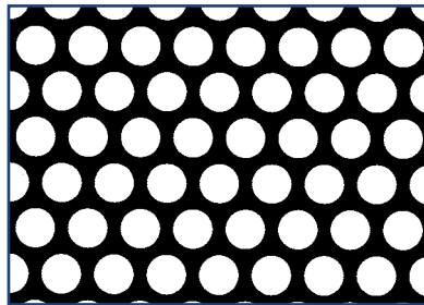
UML 105
