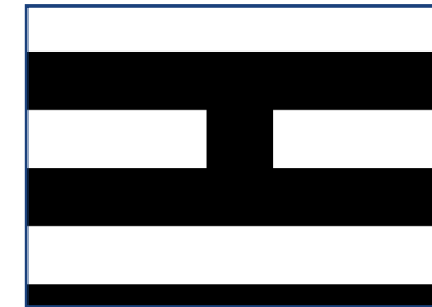
UML 120
