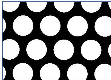
UML 111
