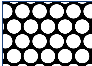
UML 109
