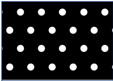
UML 104
