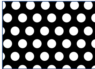
UML 106
