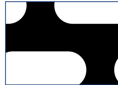
UML 119
