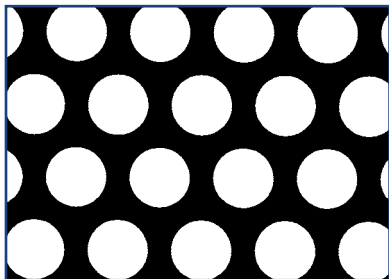
UML 110
