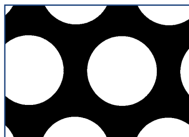
UML 115
